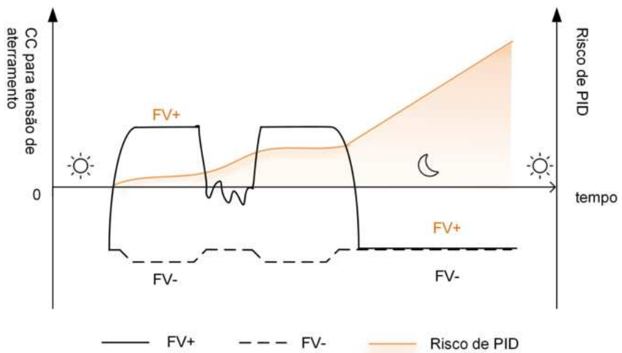
Figura 2-6 Risco de PID de inversores tradicionais
