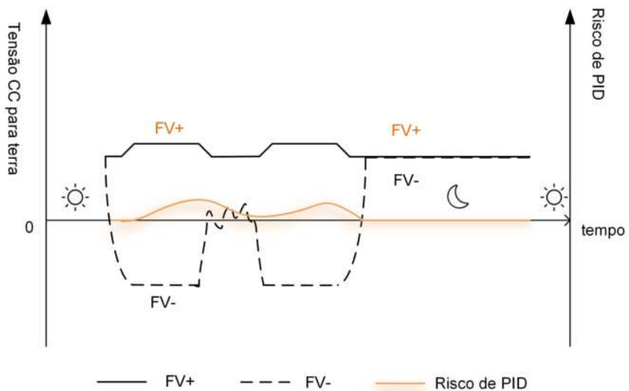
Figura 2-7 Risco de PID dos inversores equipados com Zero PID
